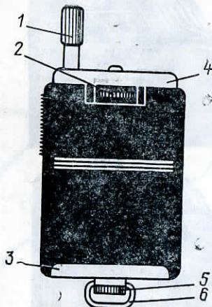
Рис. 7. Устройство приставки 1 — колпачок; 2 — винт крепления приставки к экспонометру; 3 — скоба нижняя; 4 — скоба верхняя; 5 — винт, 6 — скоба для шнура
